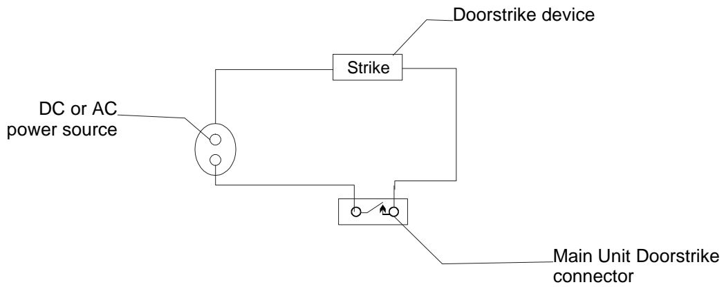
Fig 4.- Doorstrike Hook up diagram
